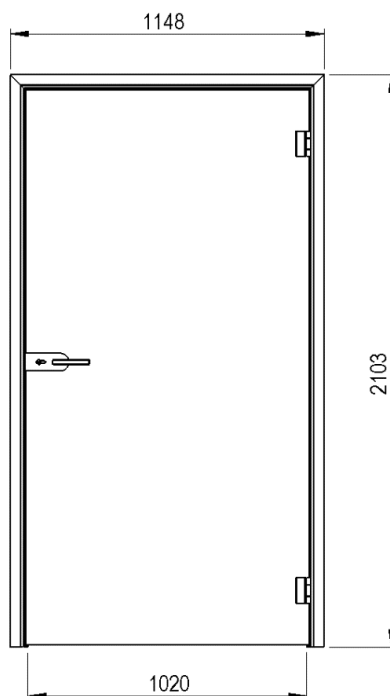
Rys. Drzwi TAW 1 (maksymalne wymiary).
