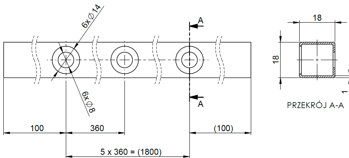
Rys. Rysunek Adaptera montażowego.
