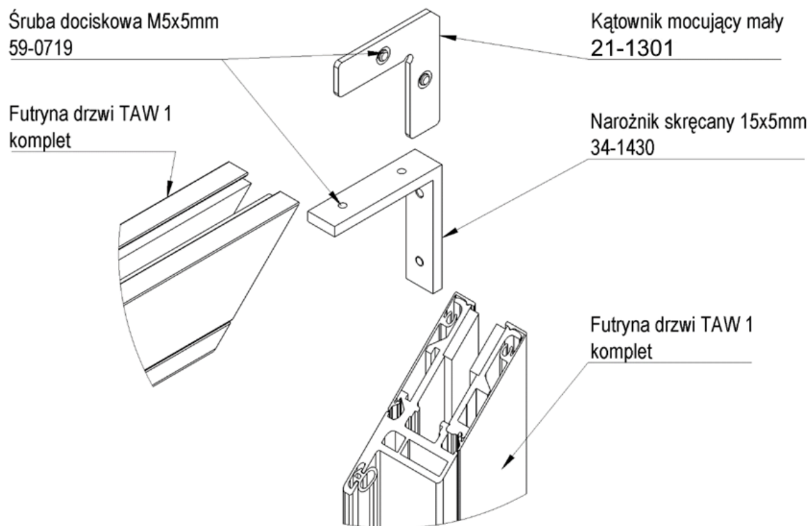
Rys. Montaż futryny drzwi.
