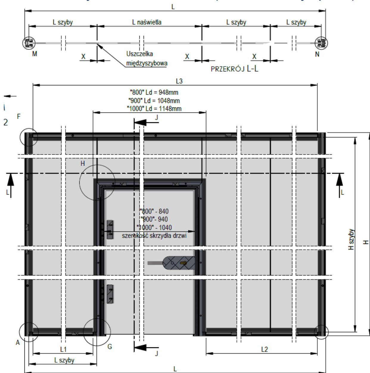
Rys. Zależności w ścianie z drzwiami.
