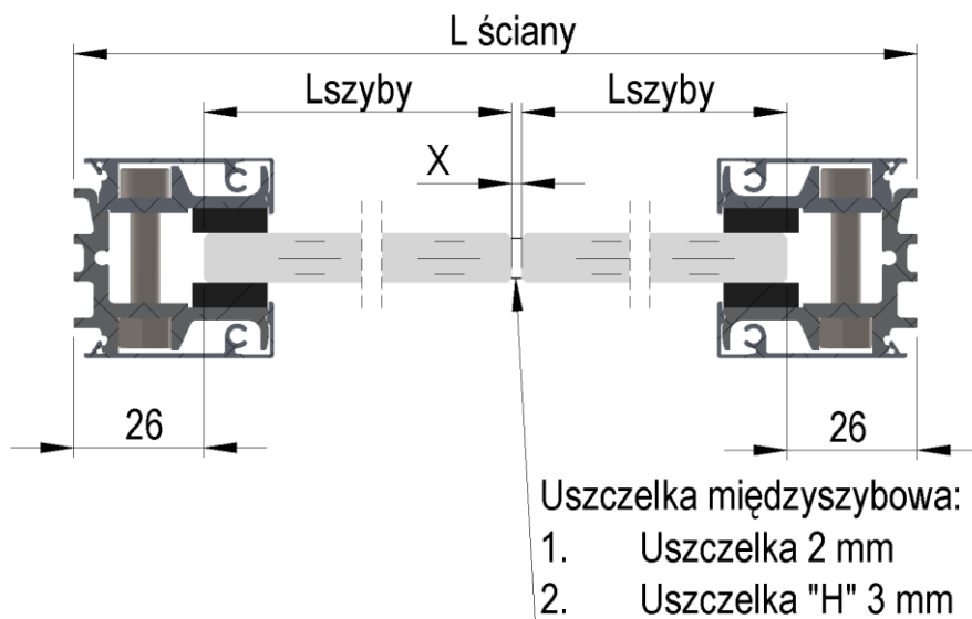
Rys. Zależności wymiarowe w panelu (przekrój poziomy).
