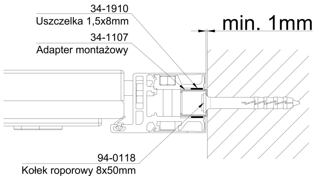
Rys. Sposób mocowania futryny drzwi do ściany za pomocą Adaptera montażowego.
