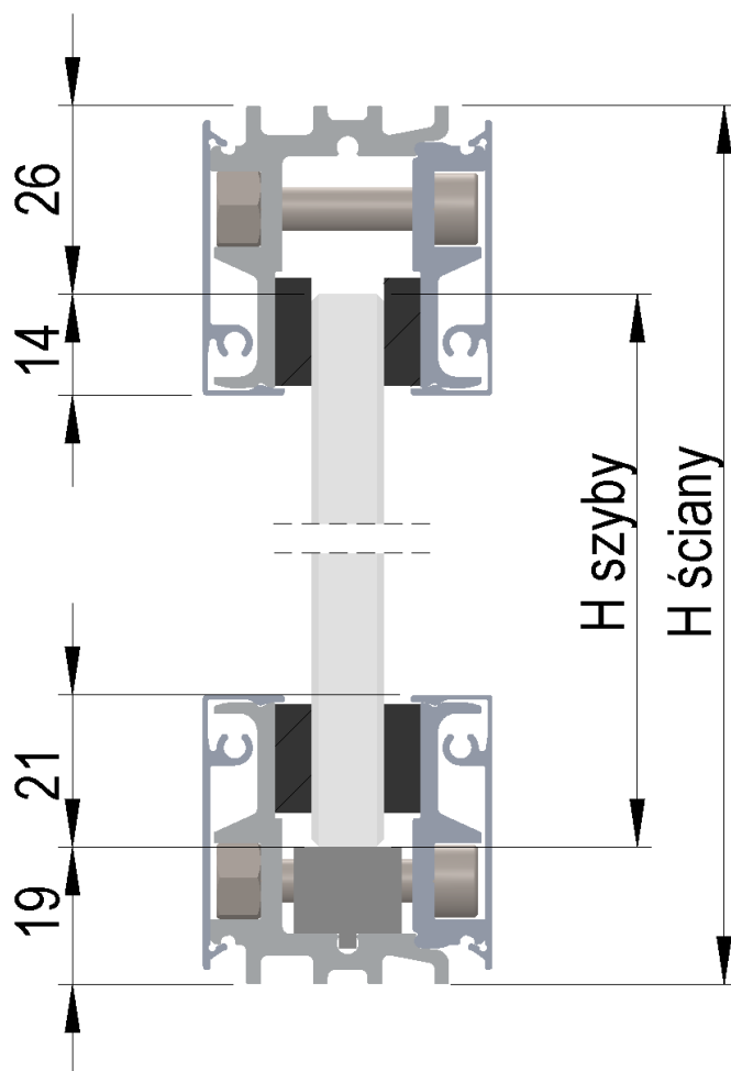
Rys. Zależności wymiarowe w panelu (przekrój pionowy).
