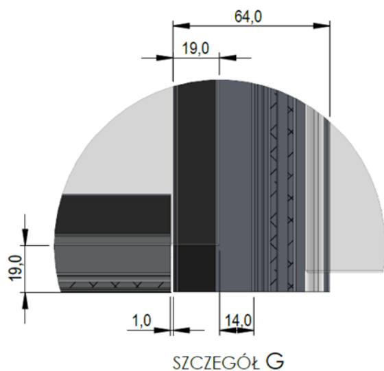
Rys. Zależności w ścianie z drzwiami.
